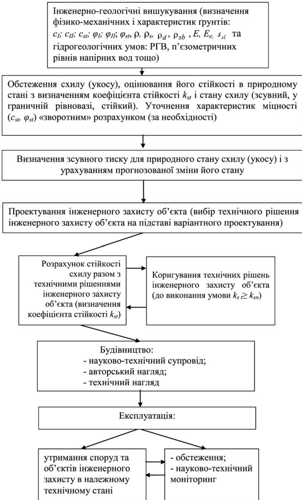
Рисунок В.1 – Основні етапи проектування, будівництва та експлуатації споруд та об'єктів інженерного захисту
