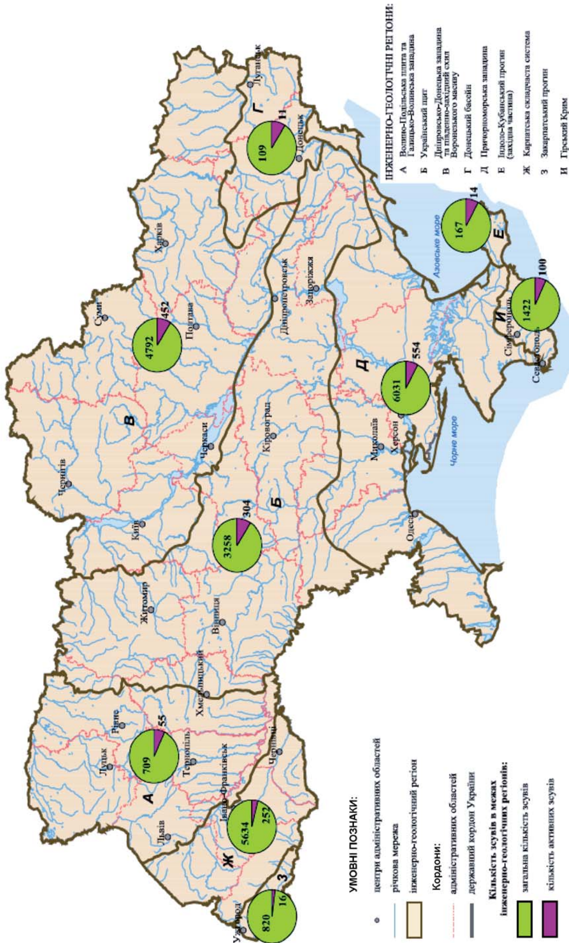
Рисунок А.2 – Поширення зсувів у межах інженерно-геологічних регіонів України
